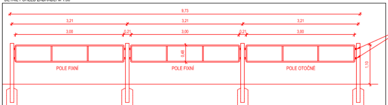
DETAIL POHLED ZÁBRADLÍ M 1:50
